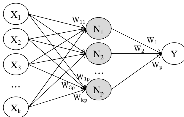
Figura 19 Representação de obtenção do escore neural
