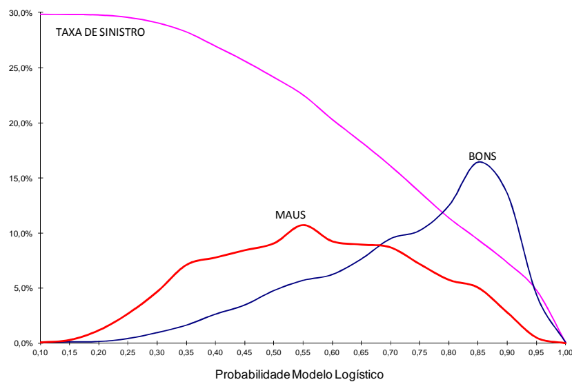
Figura 22 Distribuição dos clientes e taxa de sinistro com modelo logístico
