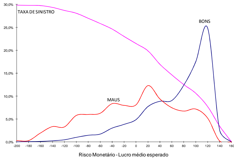
Figura 25 Distribuição dos clientes e taxa de sinistro com modelo de previsão do lucro
