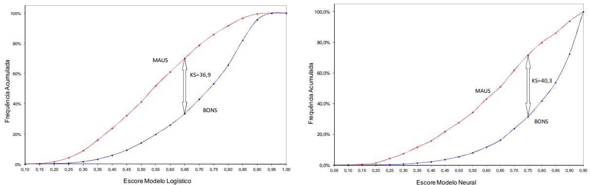
Figura 24 Representação do valor de KS para os modelos construídos
