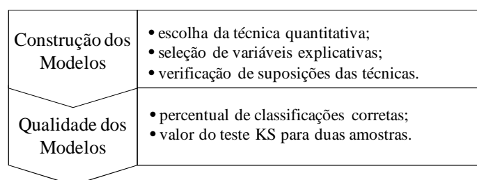
Figura 16 Etapa de obtenção dos modelos de classificação
