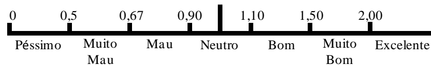
Figura 15 Classes de risco relativo para agrupamento.
