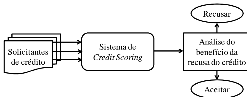
Figura 1 Processo de concessão de crédito com modelos de credit scoring
