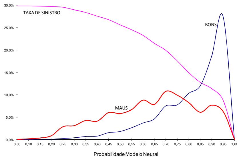
Figura 23 Distribuição dos clientes e taxa de sinistro com modelo neural
