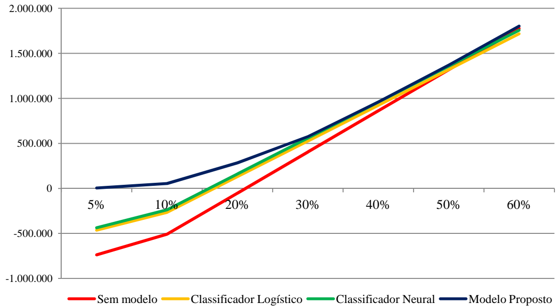
Figura 27 Análise de sensibilidade da previsão do lucro modificando a margem
