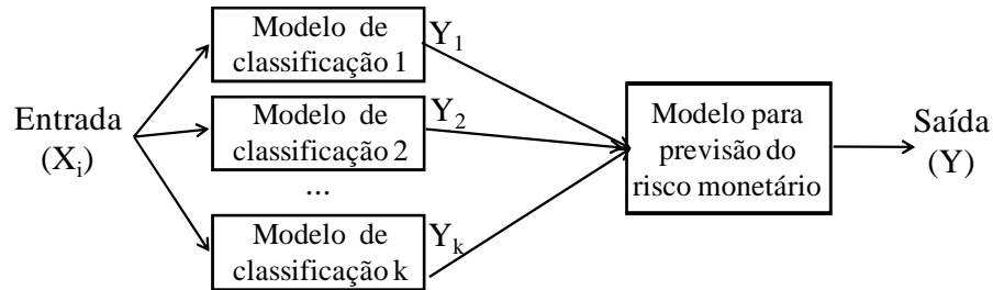
Figura 17 Esquema de análise para construção do modelo proposto
