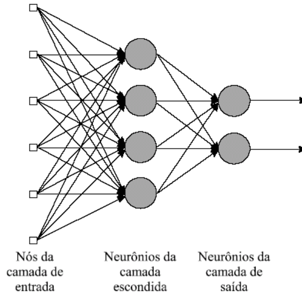
Figura 12 Modelo estrutural de uma rede neural.
