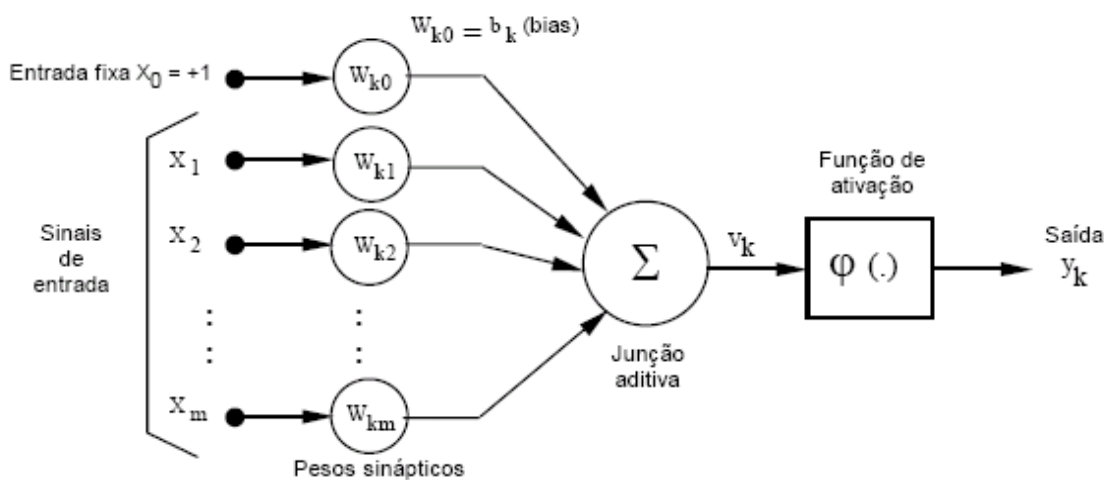
Figura 11 Modelo não linear de um nó de uma rede neural.
