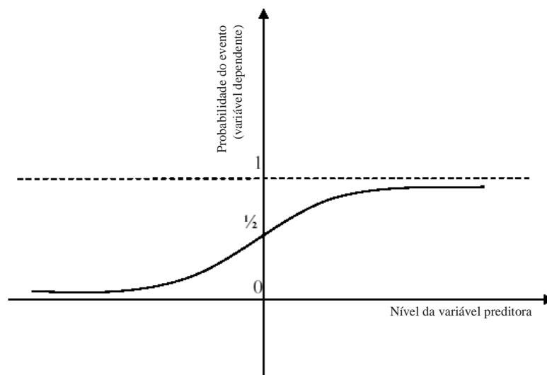
Figura 10 Forma da relação logística entre as variáveis Fonte: Hair et al. (2005)
