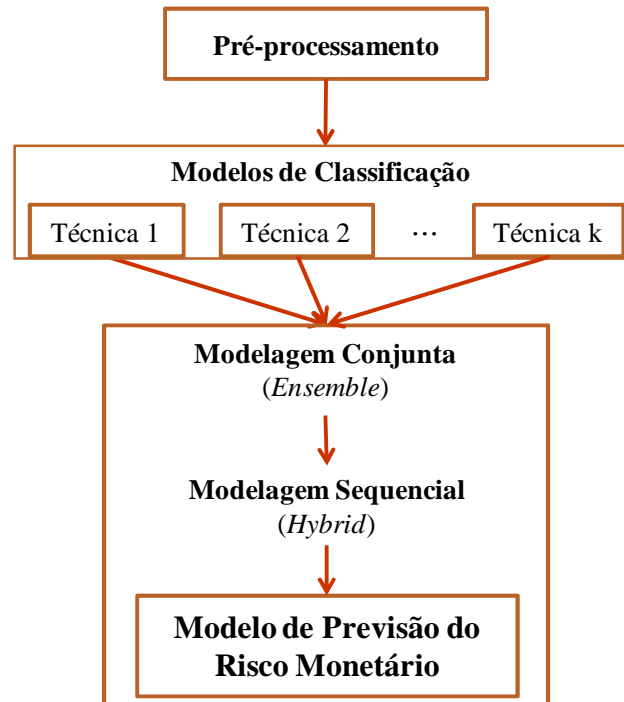
Figura 13 Modelo proposto para previsão de risco monetário
