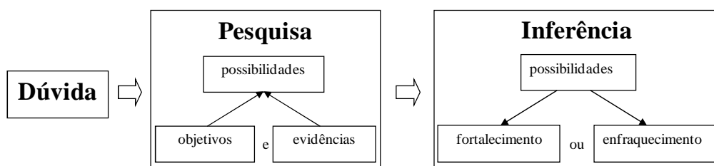
Figura 3 Estrutura de pensamento pesquisa-inferência
