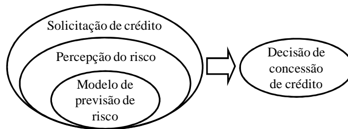
Figura 2 Relacionamento dos temas envolvidos na pesquisa
