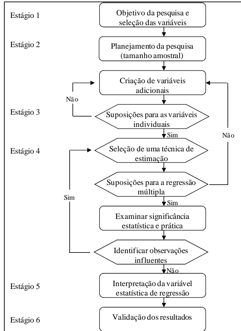
Figura 9 Processo de decisão para a regressão linear múltipla
