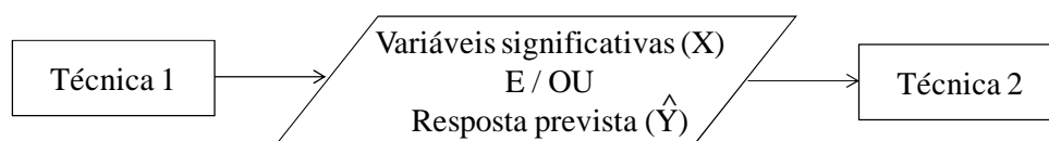
Figura 8 Representação da modelagem em sequência ( hybrid )
