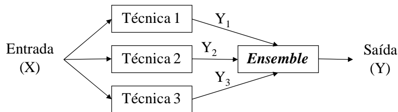
Figura 7 Representação do método de combinação de previsões ( ensemble )
