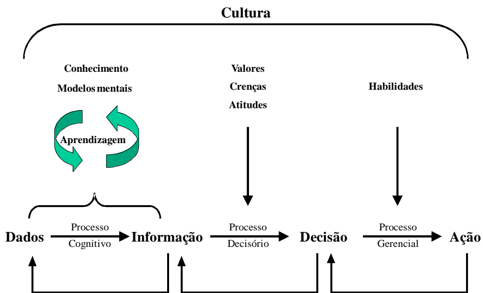
Figura 4 Influências no processo de decisão
